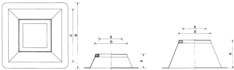
DMP/VDMP Bovenaanzicht
